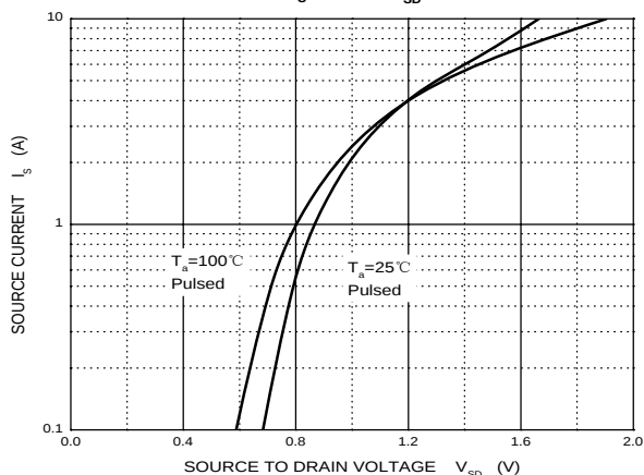
I_S — V_{SD}
